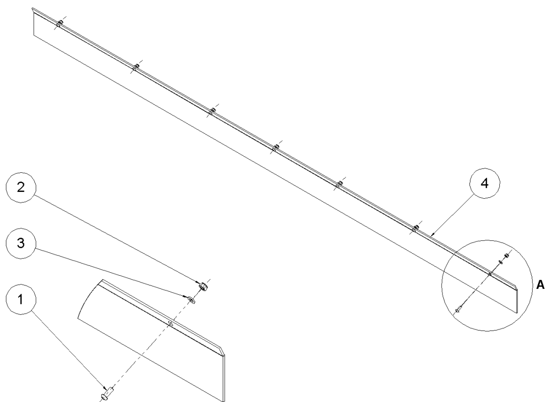
DETAIL A 2 : 7
