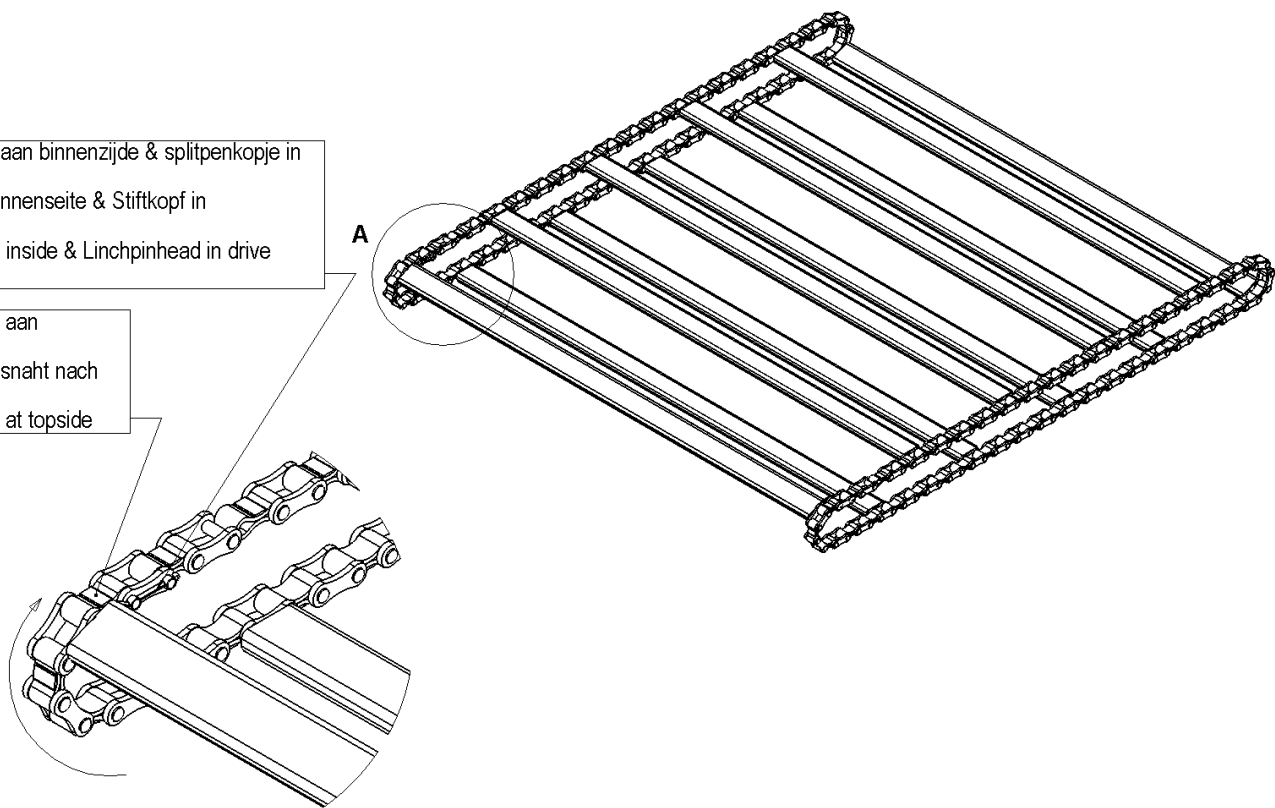
DETAIL A 1 : 5
